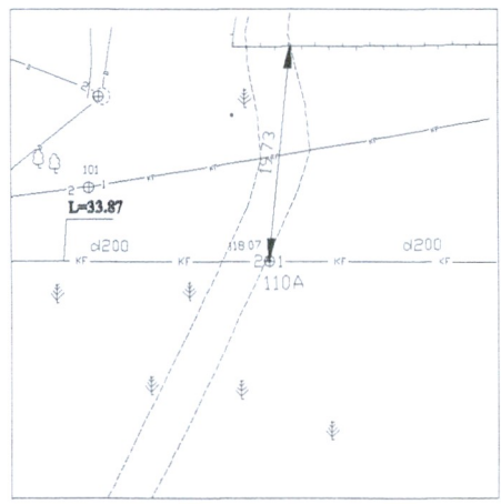
Pririšimo brėžinys:
