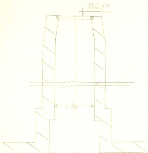
Чертеж колодца М 1:50
