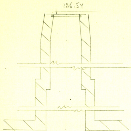
Чертеж колодца М 1:50
