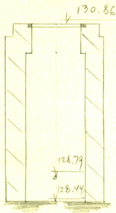
Чертеж колодца М. 1: 50
