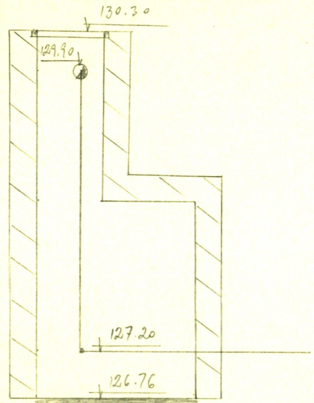
Чертеж колодца М. 1:50
