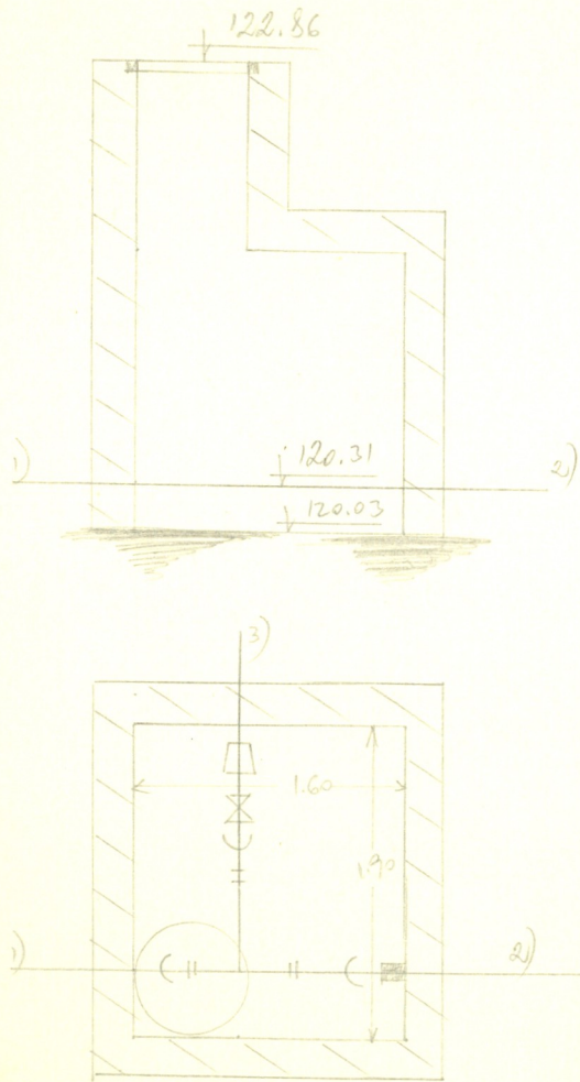
Чертеж колодца М. 1:50
