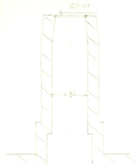
Чертеж колодца М 1:50
