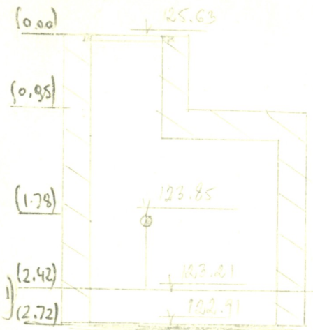
Чертеж колодца М. 1:50
