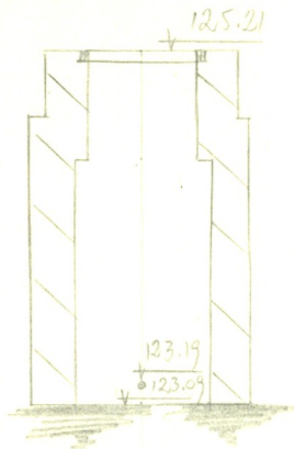
Чертеж колодца М. 1: 50
