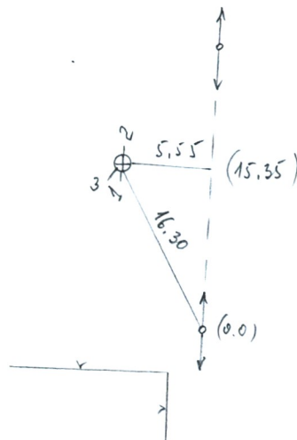
PRIRIŠIMO SCHEMA
