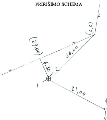
PRIRIŠIMO SCHEMA
