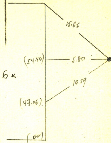
Pririšimo brėžinys:
