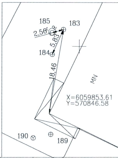
PRIRIŠIMO BRĖŽINYS
