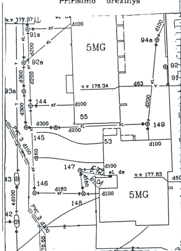
Pririšimo brėžinys
