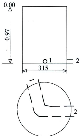
Šulinio pjūviai
