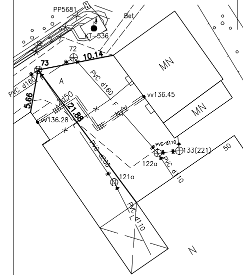
Pririšimo brėžinys
