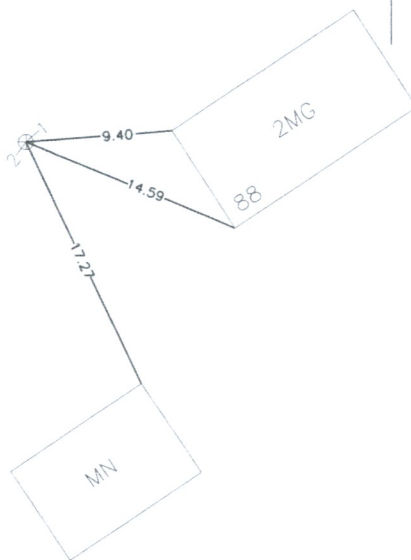
Pririšimo brėžinys
