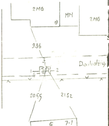
PRIRIŠIMO BRĖŽINYS
