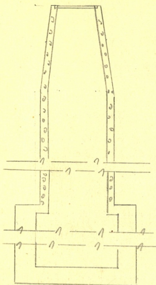
Чертеж колодца М 1:50 по А-А
