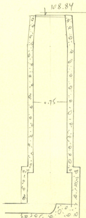
Чертеж колодца М 1:50
