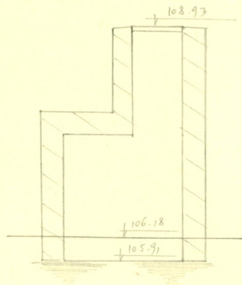
Чертеж колодца М. 1:50
