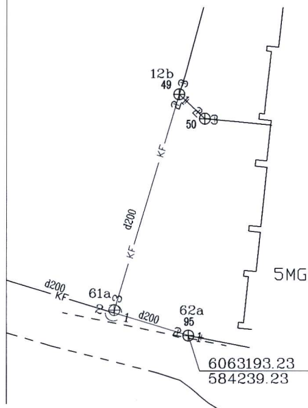
Pririšimo brėžinys
