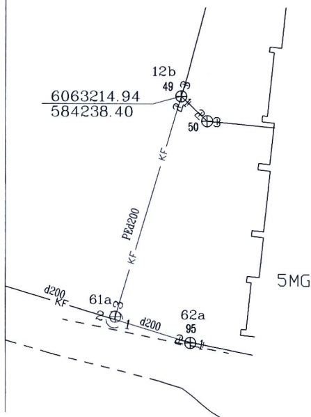
Pririšimo brėžinys
