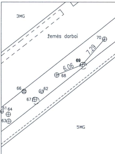
PRIRIŠIMO BRĖŽINYS
