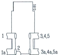
ŠULINIO PJŪVIAI (Matmenys duoti m)
