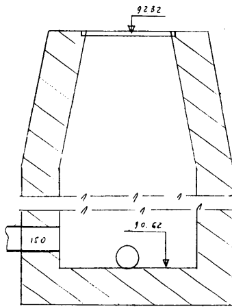
Чертеж колодца М 1:25
