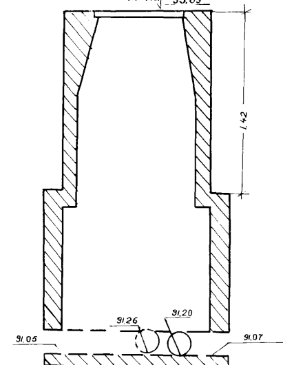
Чертеж колодца М 1:20 93.89
