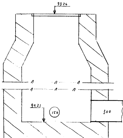
Чертеж колодца М 1:25 по А-А
