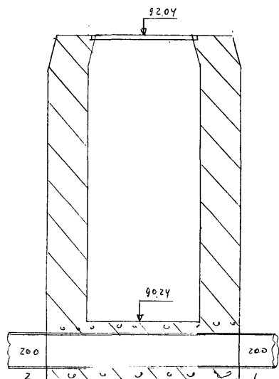
Чертеж колодца М 1:25 по А-17
