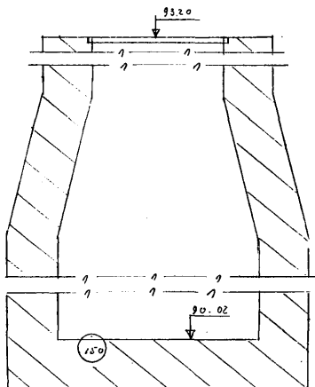
Чертеж колодца М 1:25 по А-А
