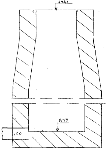
Чертеж колодца М 1:25 по А-А
