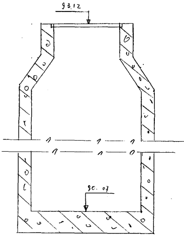
Чертеж колодца М 1:25 по А-А
