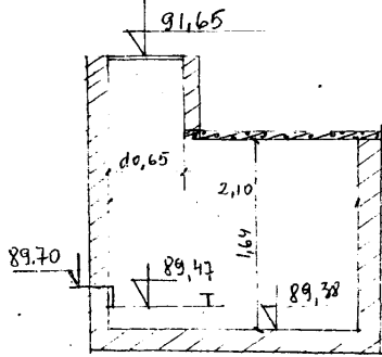
Šulinio brėžinys M 1:50
