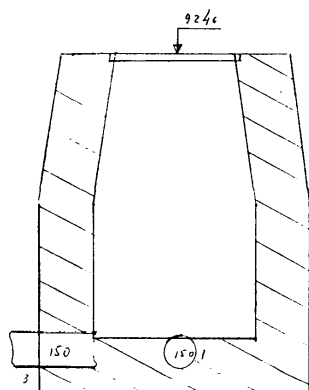
Чертеж колодца М 1:25 по А-А
