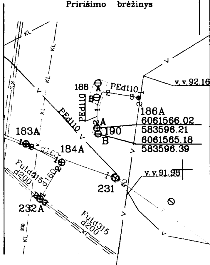
Pririšimo brėžinys
