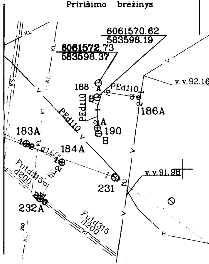
Pririšimo brėžinys
