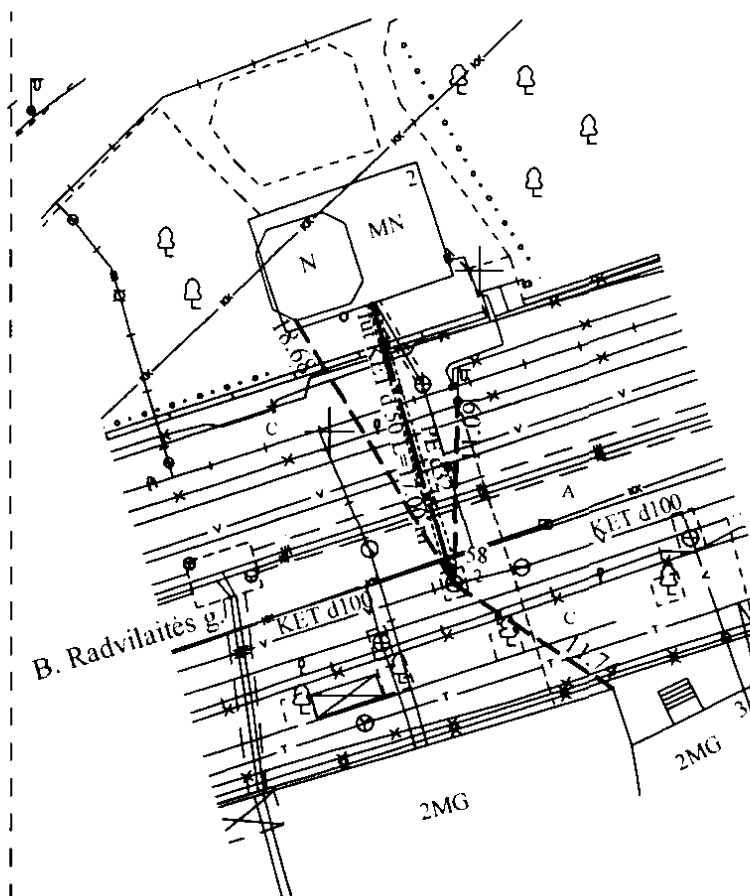
Pririšimo brėžinys
