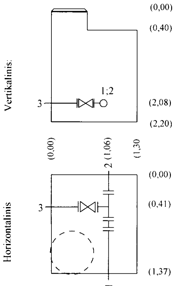
Šulinio pjūviai:
