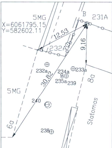
PRIRIŠIMO BRĖZINYS
