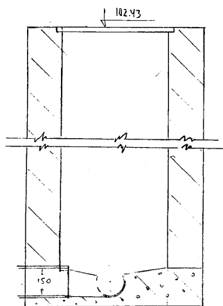
Чертеж колодца М 1:25
