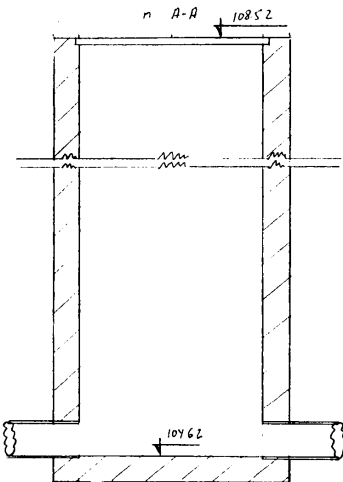
Чертеж колодца М 1:25 п. А-А
