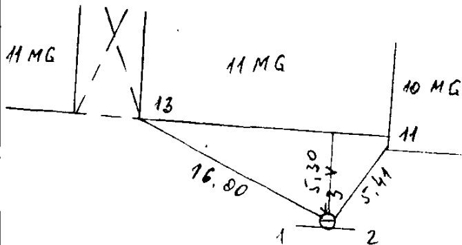
PRIRIŠIMO SCHEMA
