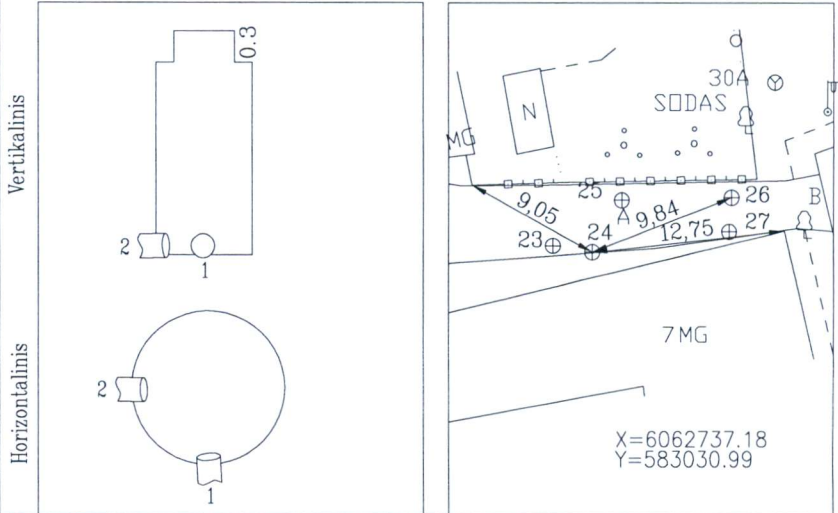
ŠULINIO PJŪVIAI (Matmenys duoti m)
