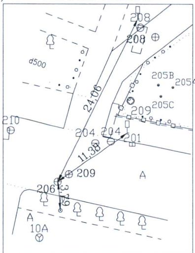
PRIRIŠIMO BRĖŽINYS
