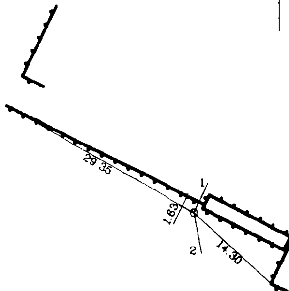
Pririšimo brėžinys
