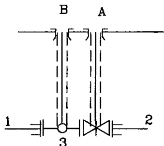
Šulinio pjūviai
