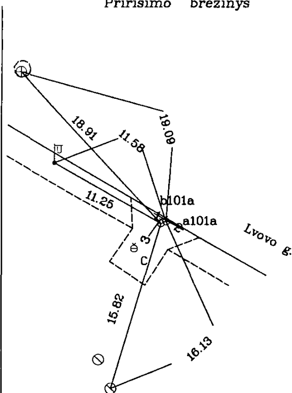
Pririšimo brėžinys
