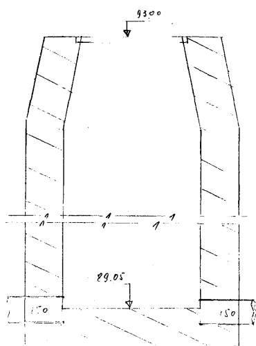
Чертеж колодца М 1:25 по 100-100
