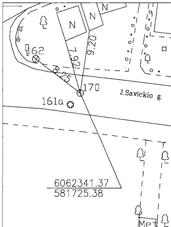
PRIRIŠIMO BRĖŽINYS
