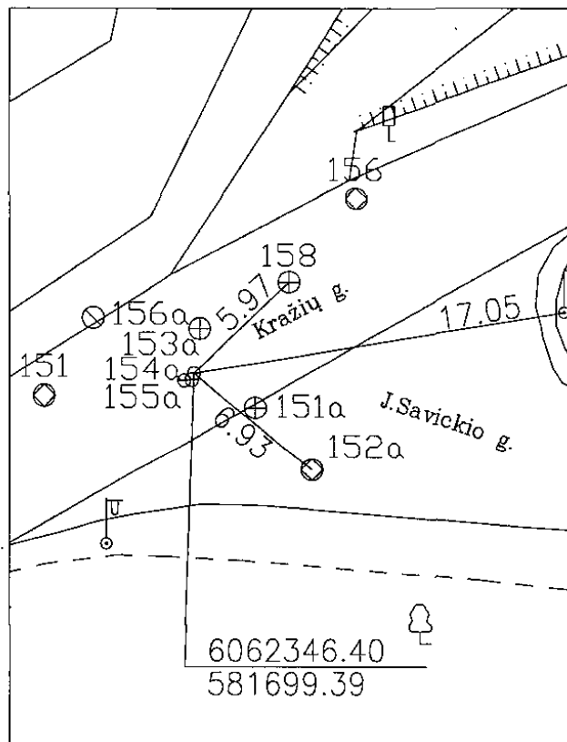
PRIRIŠIMO BRĖŽINYS
