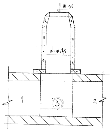
Чертеж колодца М 1:50
