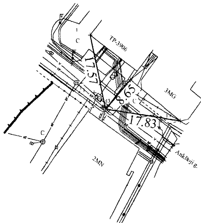
Prišimo brėžinys
